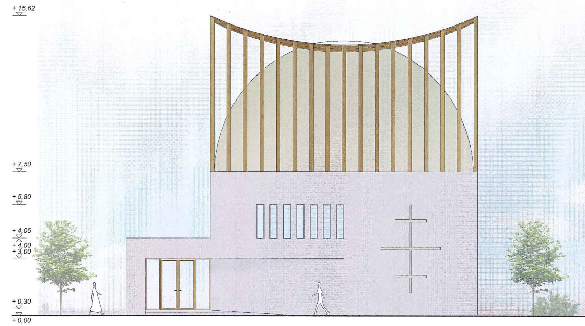
nyugati homlokzat
