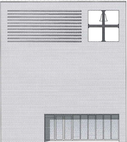
NYUGATI HOMLOKZAT
