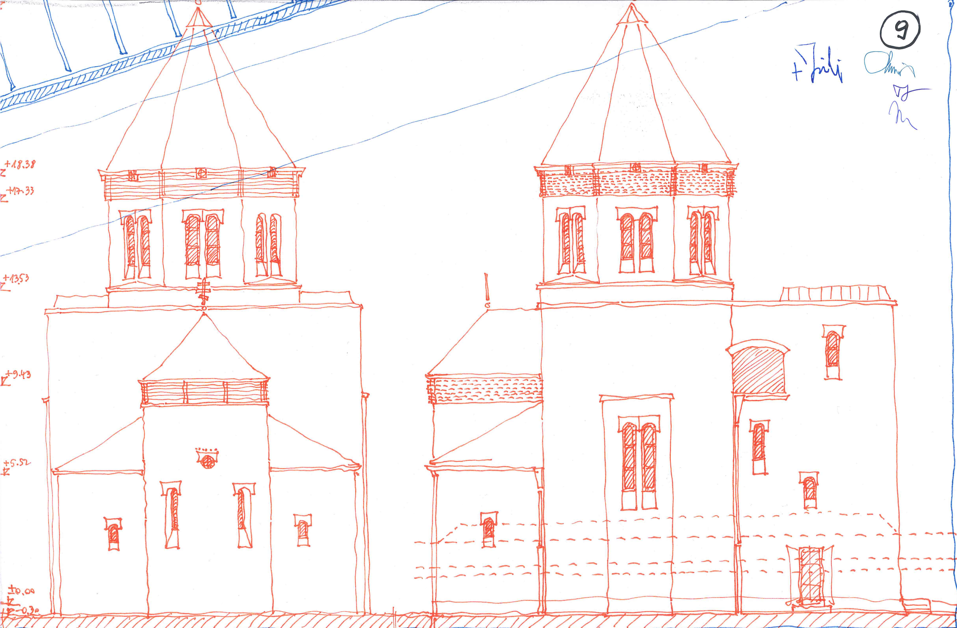
6. ⊕ DEBRECEN-TÖCÖSKERT, GÖRÖG KATOLIKUS: SZENTHÁROMSÁG: TEMPLOM: TERV PÁLYÁZAT, 2018. ⊕
